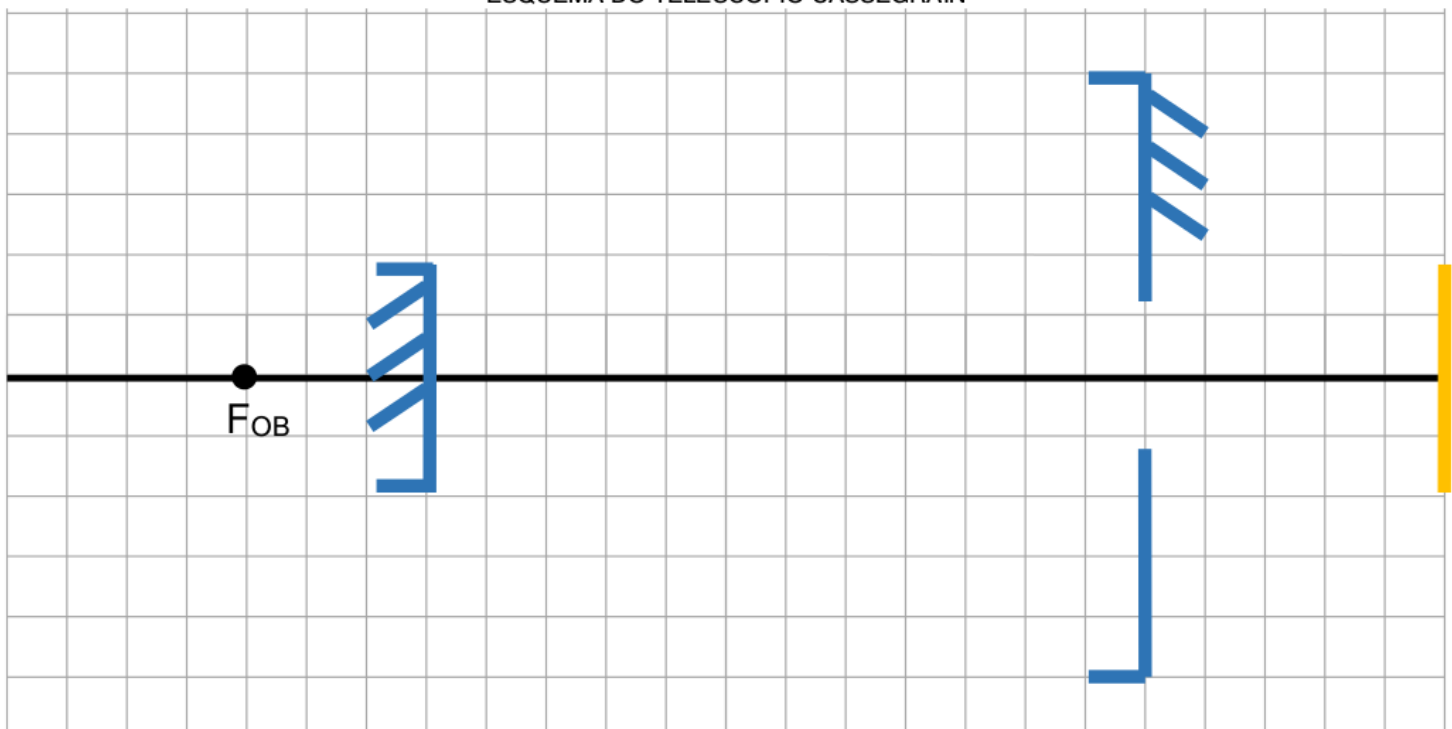
ESQUEMA DO TELESCÓPIO CASSEGRAIN
